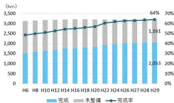
都市計画道路の整備推移（平成29年度末時点）
